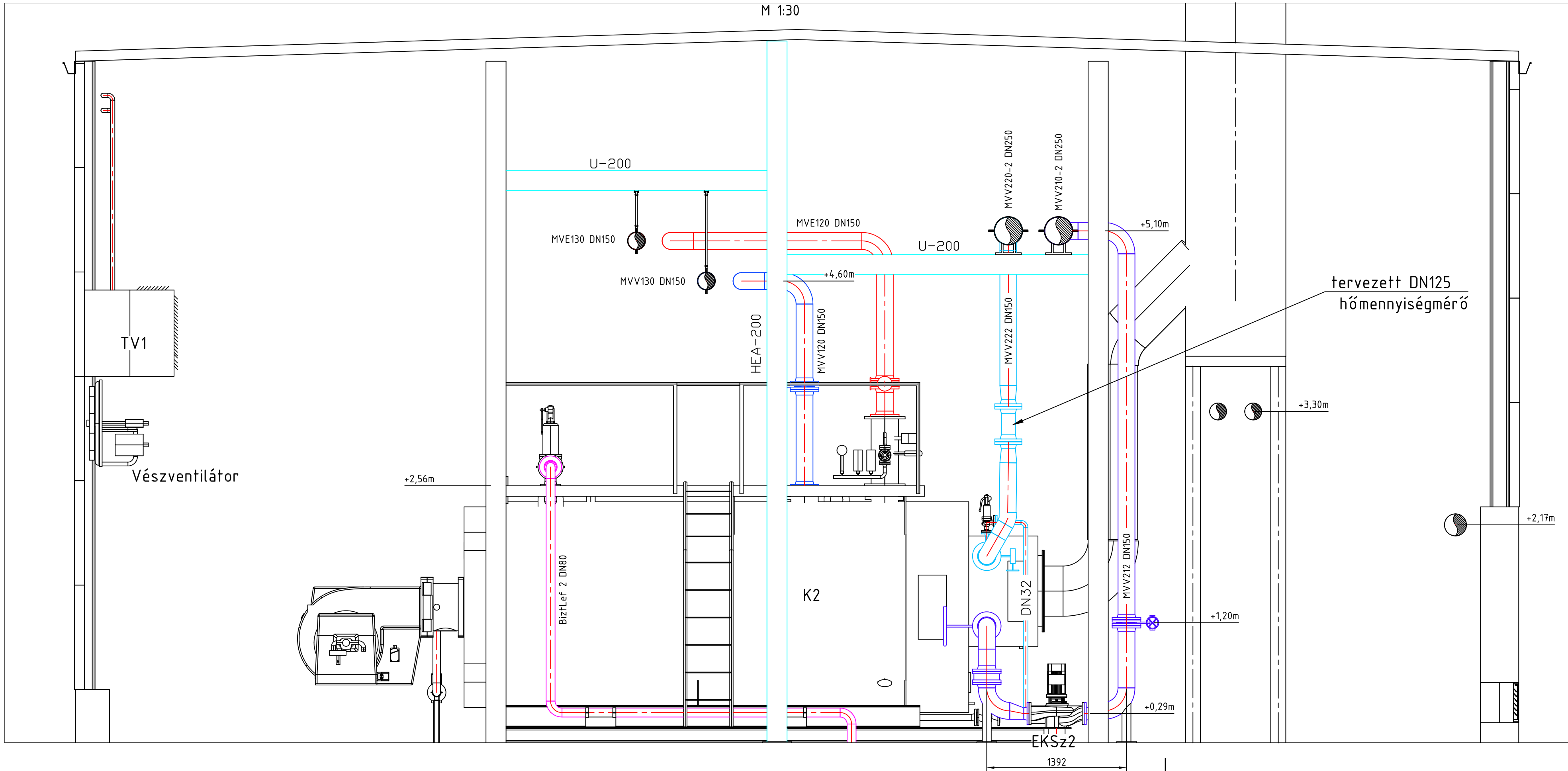
F-F metszet M 1:30
